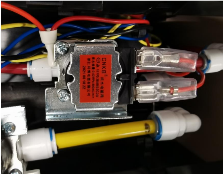
ER0265-3 （废水电磁阀）
