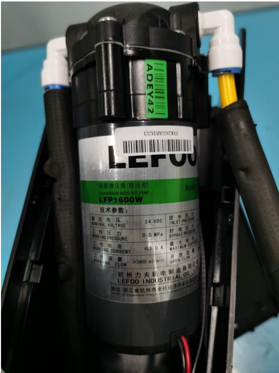
ER0265-3 （增压泵）
